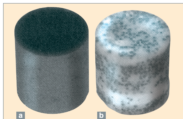
Fig. 101. pastille de combustible standard (a) et de combustible composite (b) pour la transmutation. Le combustible composite est ici composé d'une matrice inerte de spinelle (en blanc) et de macro-masses de composé d'oxyde d'actinides (en noir).
