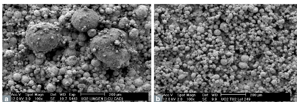
Fig. 10. Photographies au MEB montrant des agglomérats de poudres UO_2 voie sèche comparés à ceux de la poudre d' UO_2 TU2. a. Poudre d' UO_2 voie sèche (AREVA ANF) - b. Poudre d' UO_2 voie humide TU2.
