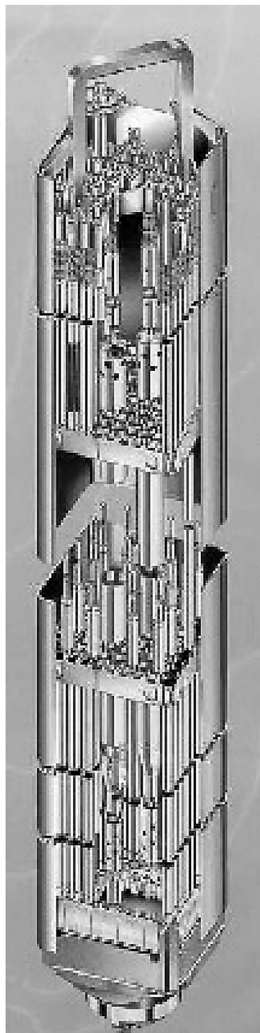
Fig. 7. Schéma d'un assemblage combustible REB.
