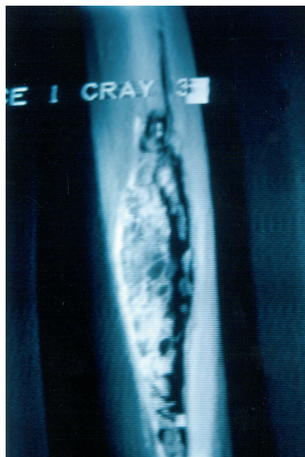
Fig. 21. Défaut d'étanchéité créé par hydruration.
