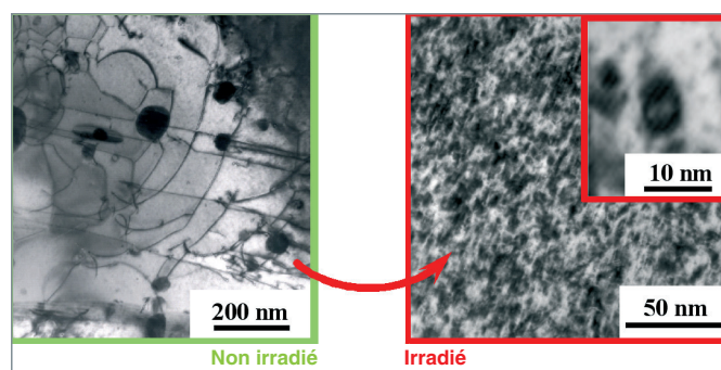
Fig. 34. Images en microscopie électronique d'un alliage de zirconium avant et après irradiation.
