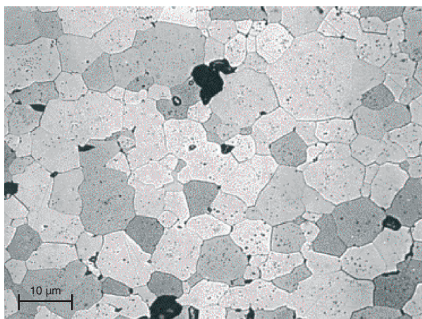
Fig. 8. Micrographie d'une céramique UO_2 après attaque chimique révélant les grains.
