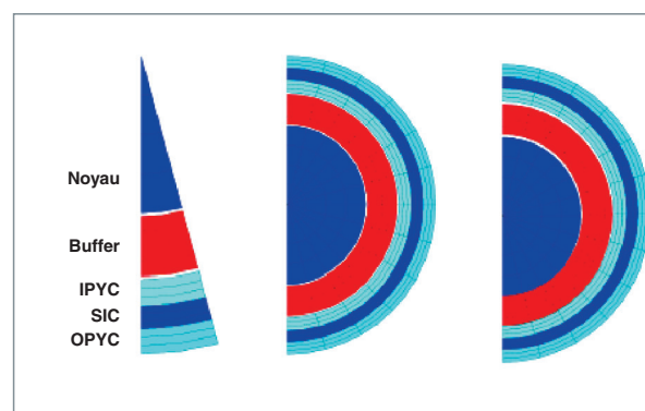
Fig. 116. Exemples de modèles d'éléments finis pour la modélisation mécanique du combustible à particules avec l'application ATLAS développée au CEA (modèle 1D, 2D centré, 2D excentré).
