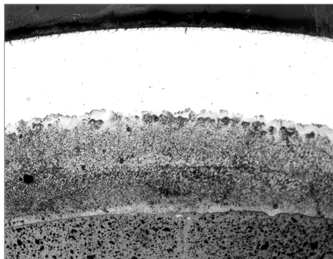
Fig. 96. Exemple d'une très importante corrosion interne de la gaine (~ 40% de l'épaisseur initiale) pour un élément combustible expérimental PHÉNIX à gaine en acier 15-15 Ti \epsilon irradié à un taux de combustion élevé (16,9 % FIMA), correspondant à une dose de 155 dpa.
