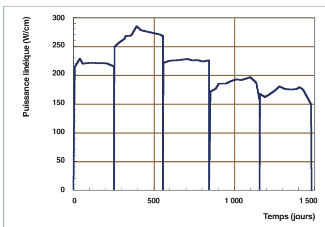
Fig. 13. Exemple d'évolution en fonction du temps de la puissance linéique moyenne d'un crayon UO_2 irradié 5 cycles dans un réacteur à eau pressurisée.
