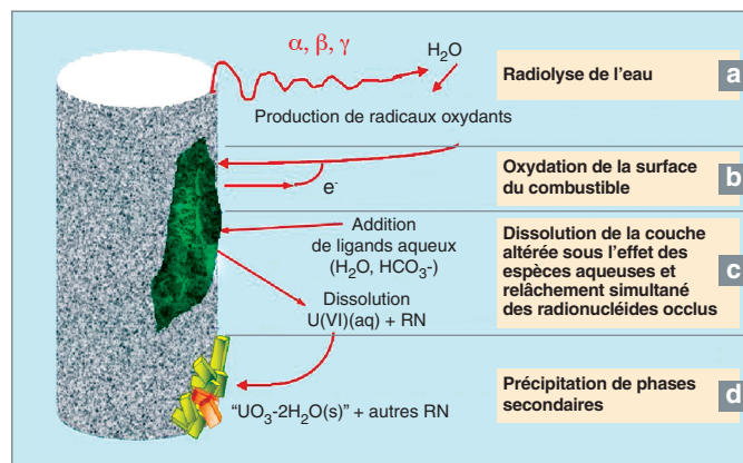
Fig. 90. Mécanismes généraux d'altération d'un combustible nucléaire usé en présence d'eau : (a) radiolyse de l'eau sous l'effet des rayonnements \alpha \beta ou \gamma , (b) oxydation de la surface du combustible et transformation de U(IV) en U(VI), (c) dissolution de la couche altérée sous l'effet des espèces aqueuses et relâchement simultané des radionucléides occlus, (d) précipitation le cas échéant de phases secondaires.
