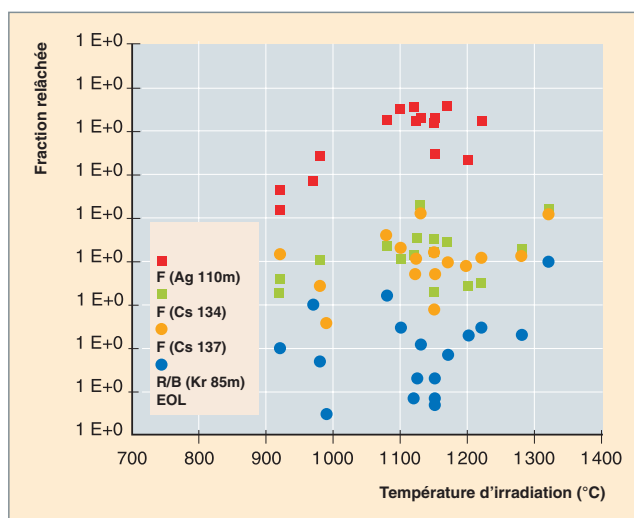
Fig. 114. Taux de relâchement de différents types de produits de fission : gazeux (krypton), volatil (Césium) et métallique (argent) en fonction de la température d'irradiation pour des particules \text{UO}_2 à faible enrichissement en U 235 TRISO dans des boulets allemands.
