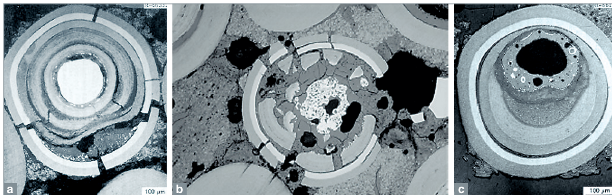
Fig. 111. Différents modes de ruine des particules. a) : Accumulation de PF ; b) : Suppression ; c) : Effet amibe L'effet amibe correspond au déplacement du noyau dans le buffer dû à un transport des atomes de carbone du buffer du côté chaud vers le côté froid à
