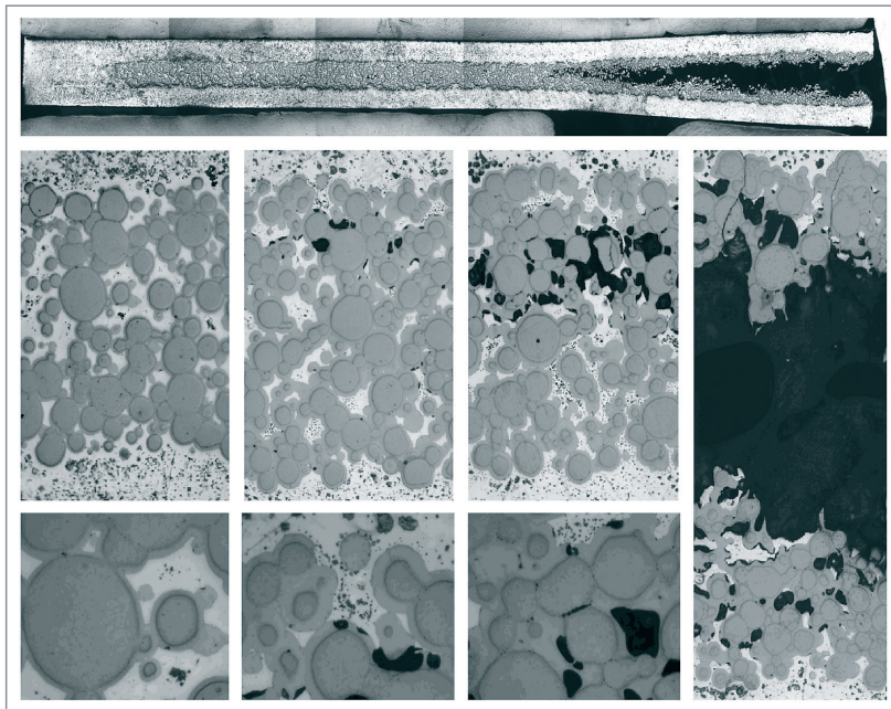
Fig. 128. Examens métallographiques réalisés au plan de flux maximal d'une plaque IRIS2 irradiée.
