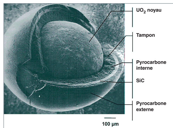
Fig. 104. Fractographie d'une particule \text{UO}_2 -TRISO-SiC.
