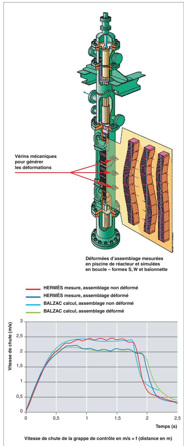
Fig. 52. Schéma du dispositif expérimental dédié à la mesure de cinétique de chute pour différentes déformations de l'assemblage combustible.
