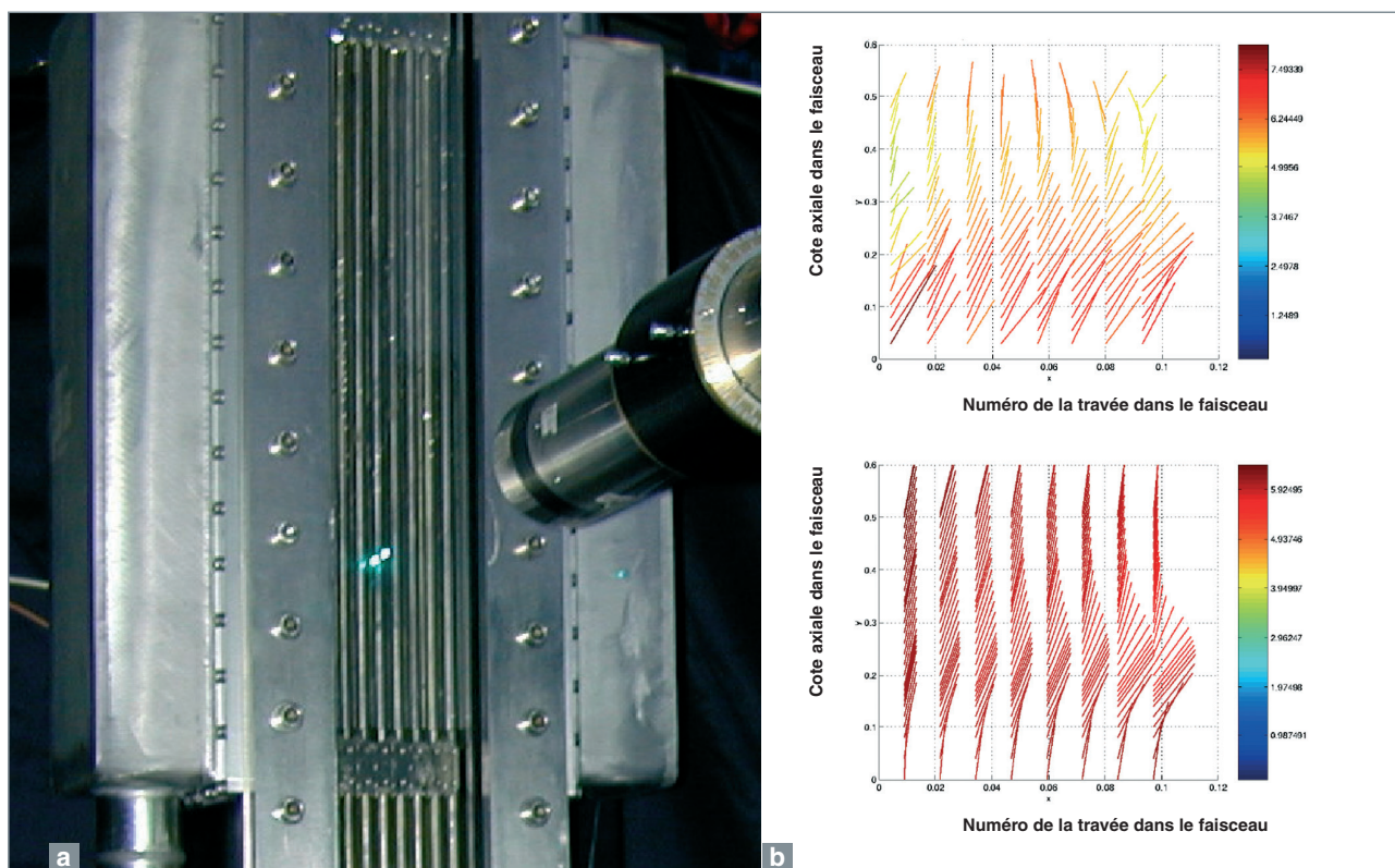
Fig. 50. Photo du banc de vélocimétrie laser installé sur le dispositif expérimental dédié à la caractérisation des écoulements et aux mesures des efforts sur le faisceau combustible (a).
