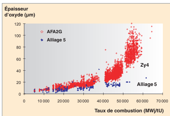
Fig. 39. Épaisseurs d'oxyde sur crayons Zy-4 avec combustible UO_2 [6]. On observe une accélération de la corrosion pour les taux de combustion élevés ou les temps de séjour longs. Le gain apporté par le nouvel alliage M5 ® apparaît clairement.
